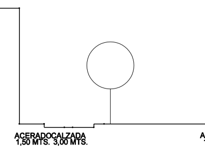
VIARIO V4. ANCHO TOTAL = 24,00 MTS.
